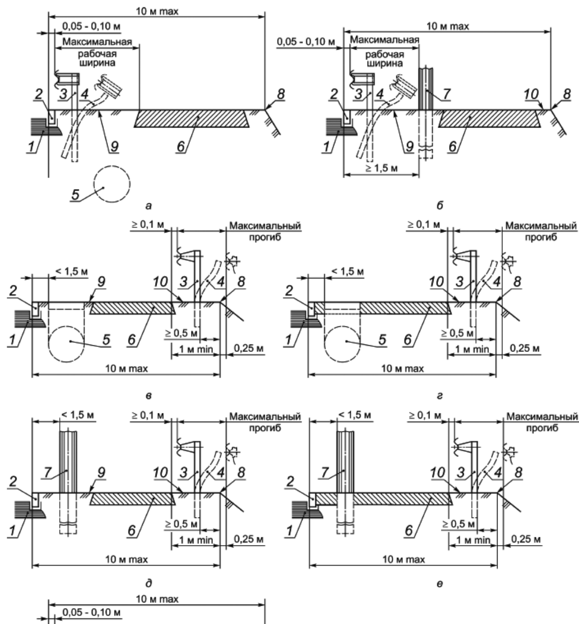
Рисунок В.28 - Примеры установки дорожных ограждений
