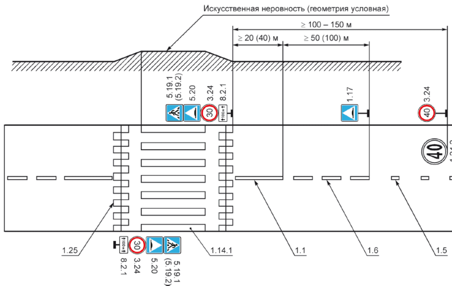
Рисунок В.20 - Пример размещения светофоров и нанесения разметки на регулируемом переходе
