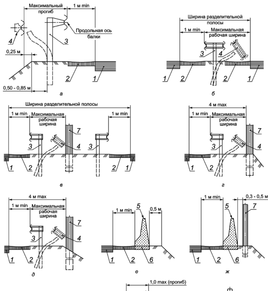
Рисунок В.27 - Смещение дорожного ограждения
