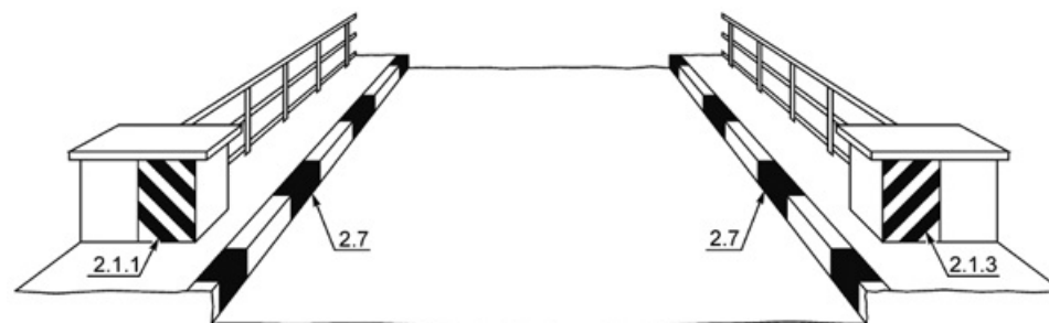
Рисунок В.22 - Пример нанесения разметки 2.1 и 2.2
