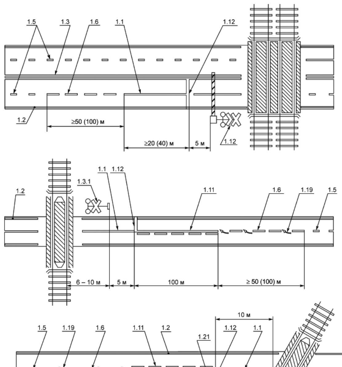
Рисунок В.17 - Примеры нанесения разметки 1.9
