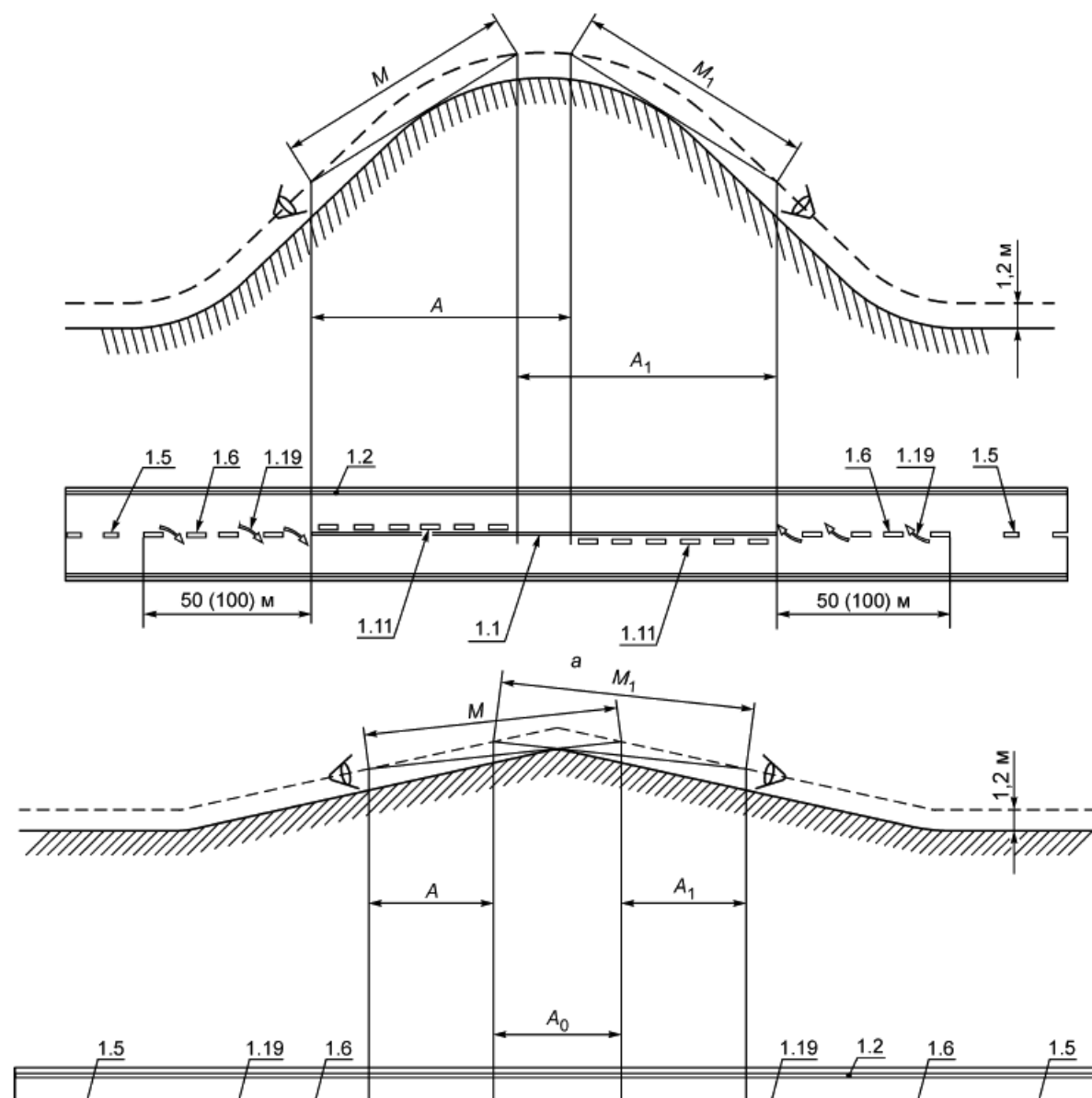
Рисунок В.5 - Пример расстановки знаков 5.1 и 5.2
