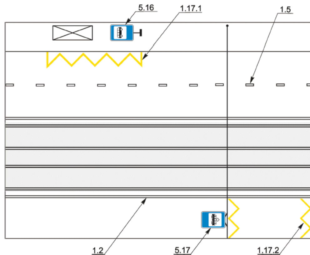
Рисунок В.14 - Пример нанесения разметки в местах остановки маршрутных транспортных средств
