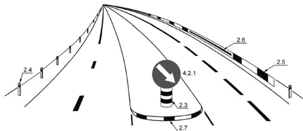
Рисунок В.23 - Пример нанесения разметки 2.1.1, 2.1.3 и 2.7
