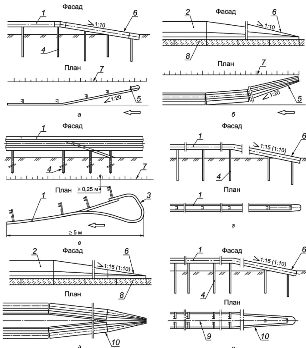
Рисунок В.29 - Примеры установки дорожных ограждений
