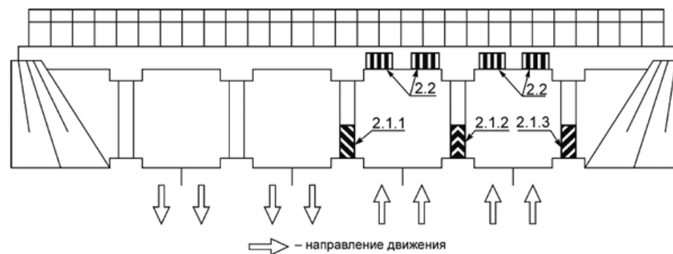
Рисунок В.21 - Пример нанесения разметки 1.25
