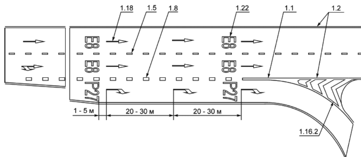
Рисунок В.15 - Пример нанесения разметки 1.17.1 и 1.17.2
