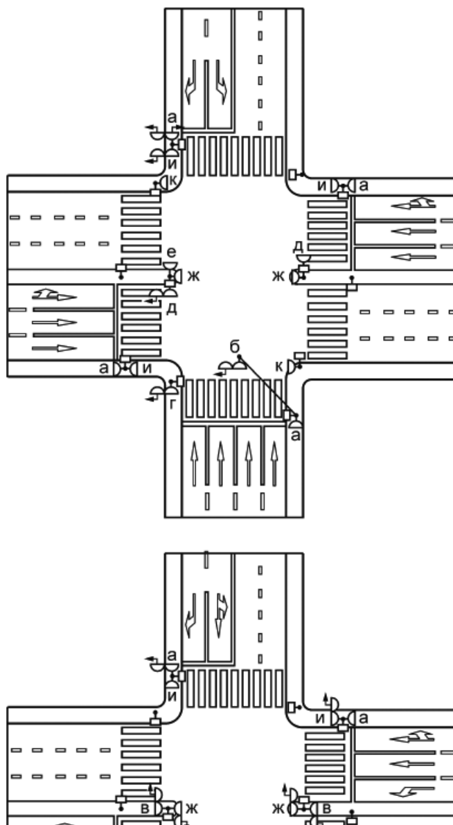
Рисунок В.25 - Примеры установки светофоров различных типов и исполнений
