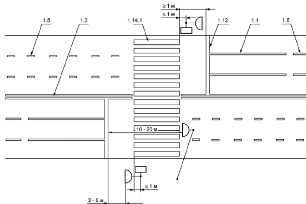
Рисунок В.19 - Пример нанесения диагонального пешеходного перехода
