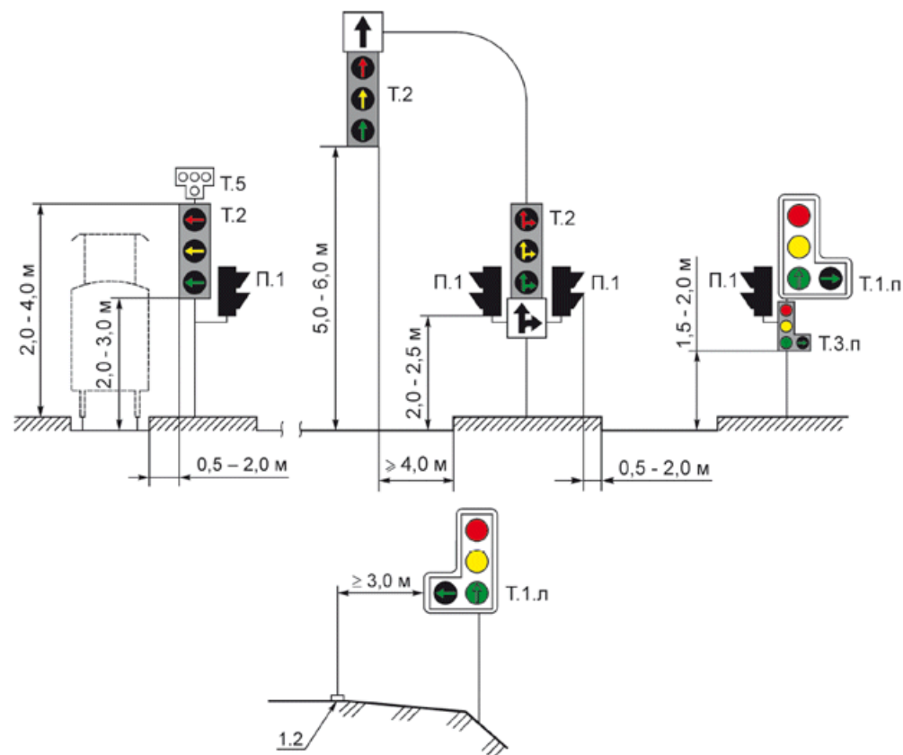
Рисунок В.24 - Пример нанесения разметки 2.3-2.7
