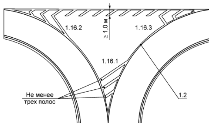
Рисунок В.11 - Пример разметки участка дороги со специальной полосой для маршрутных транспортных средств
