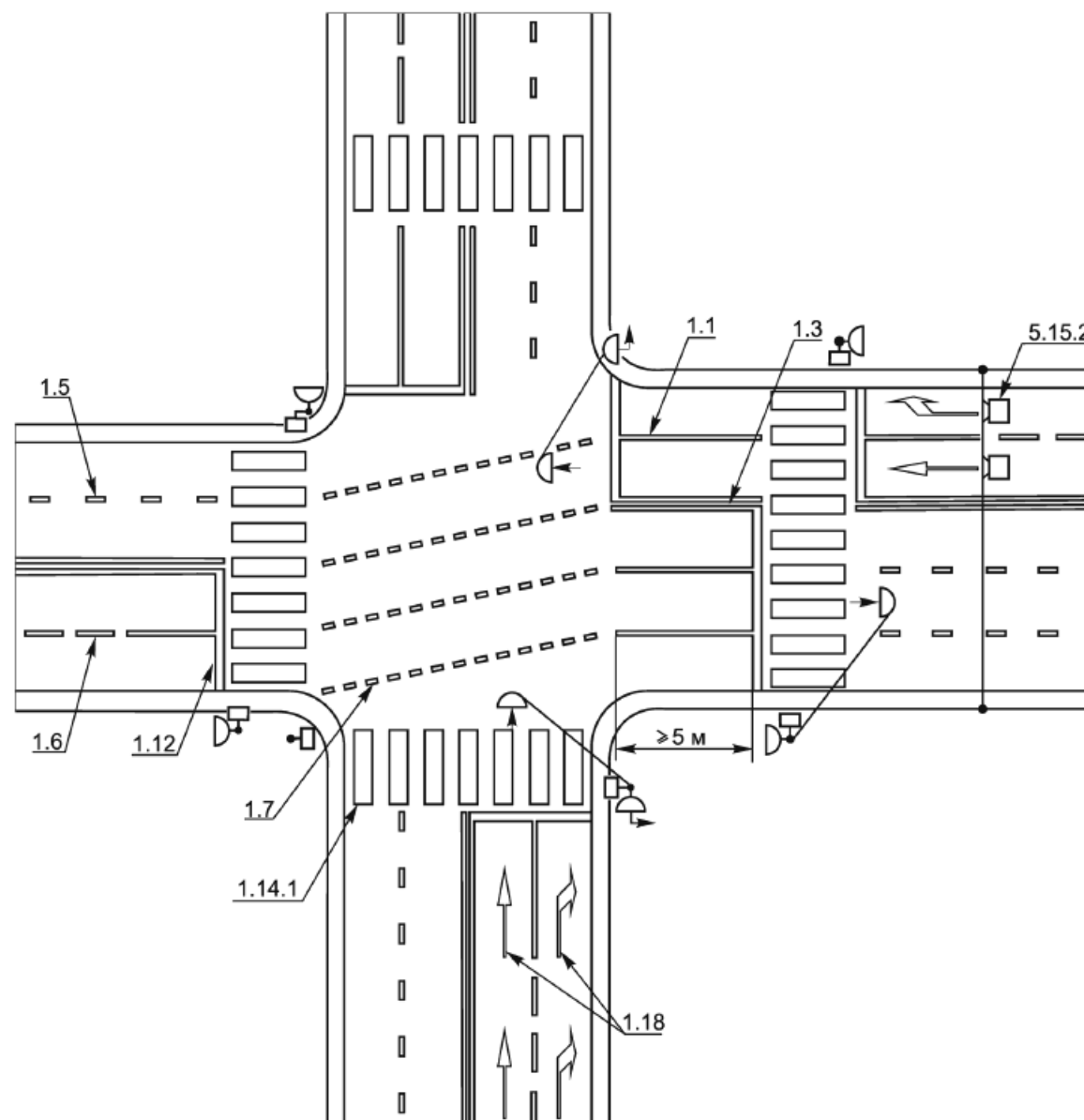
Рисунок В.8 - Пример нанесения разметки при уменьшении и увеличении количества полос для движения в одном направлении
