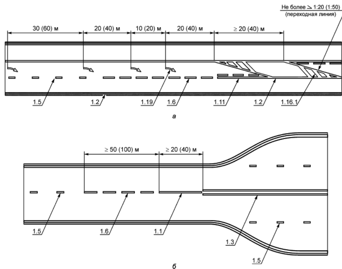
Рисунок В.7 - Пример нанесения разметки перед нерегулируемым перекрестком с ограниченной видимостью
