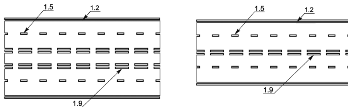
Рисунок В.16 - Пример нанесения разметки на участке съезда с автомагистрали
