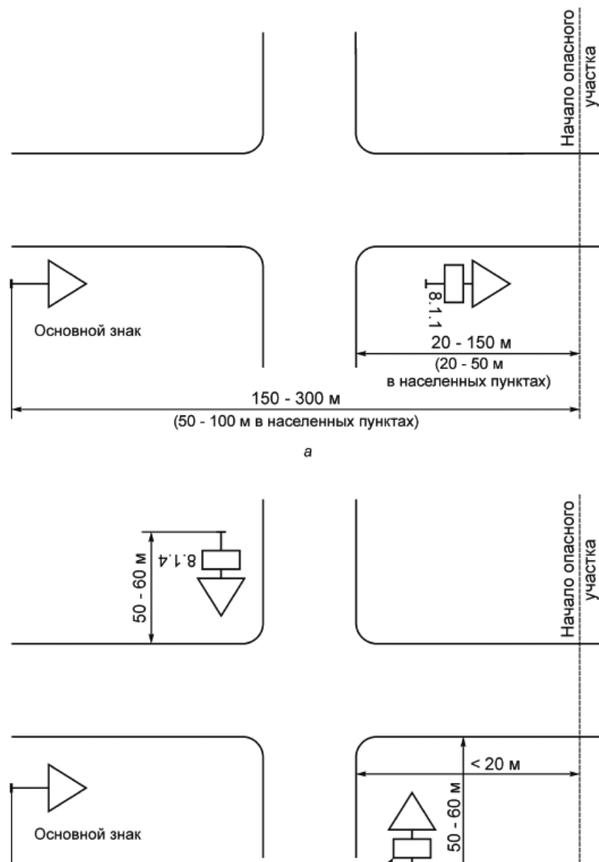
Рисунок В.1 - Типовое размещение знаков в поперечном профиле дороги
