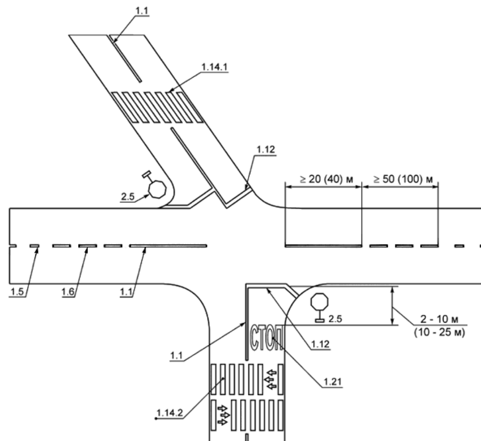
Рисунок В.6 - Примеры нанесения разметки на участках дорог с необеспеченной видимостью в зависимости от зоны видимости встречного автомобиля
