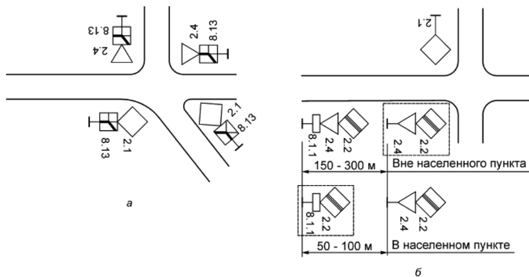
Рисунок В.3 - Размещение знаков 1.4.1-1.4.6
