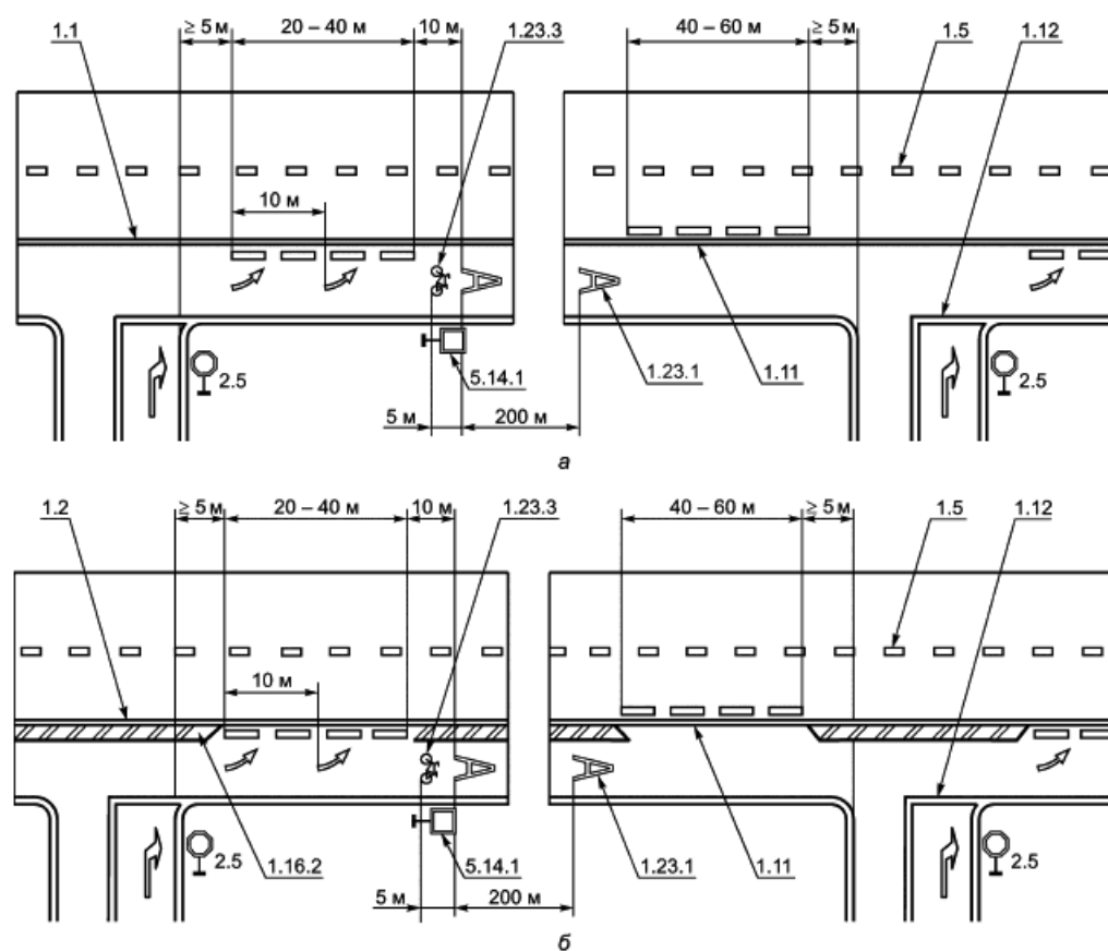
Рисунок В.10 - Пример нанесения разметки канализированного пересечения
