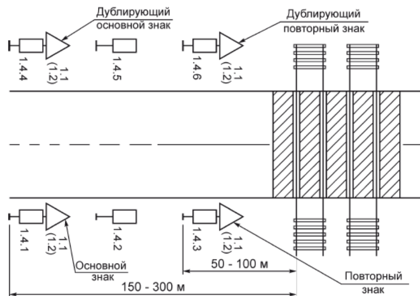
Рисунок В.2 - Установка предупреждающих знаков
