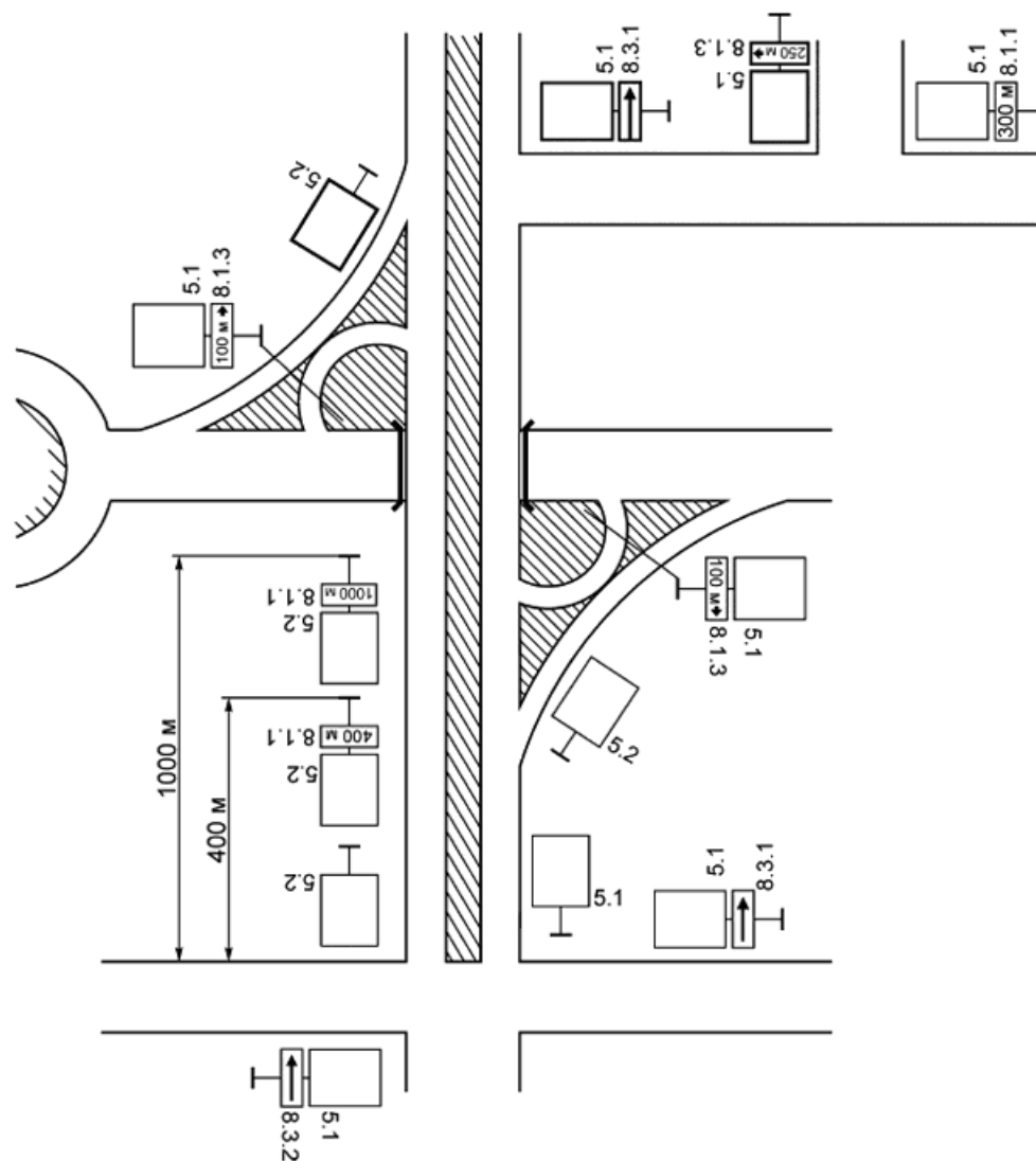
Рисунок В.4 - Размещение знаков приоритета
